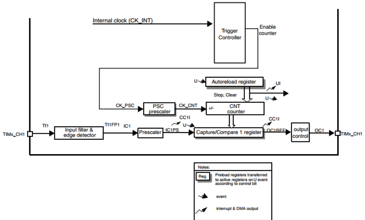
图 16-1 TIMx(TIM10/TIM11/TIM13/TIM14)模块
