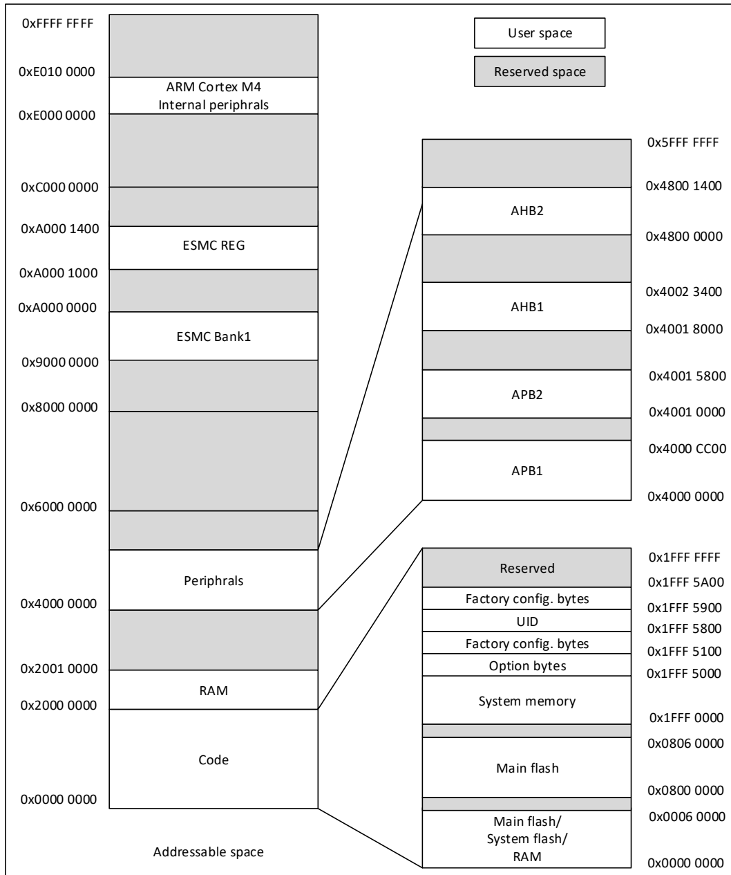
图 2-2 存储器映射
